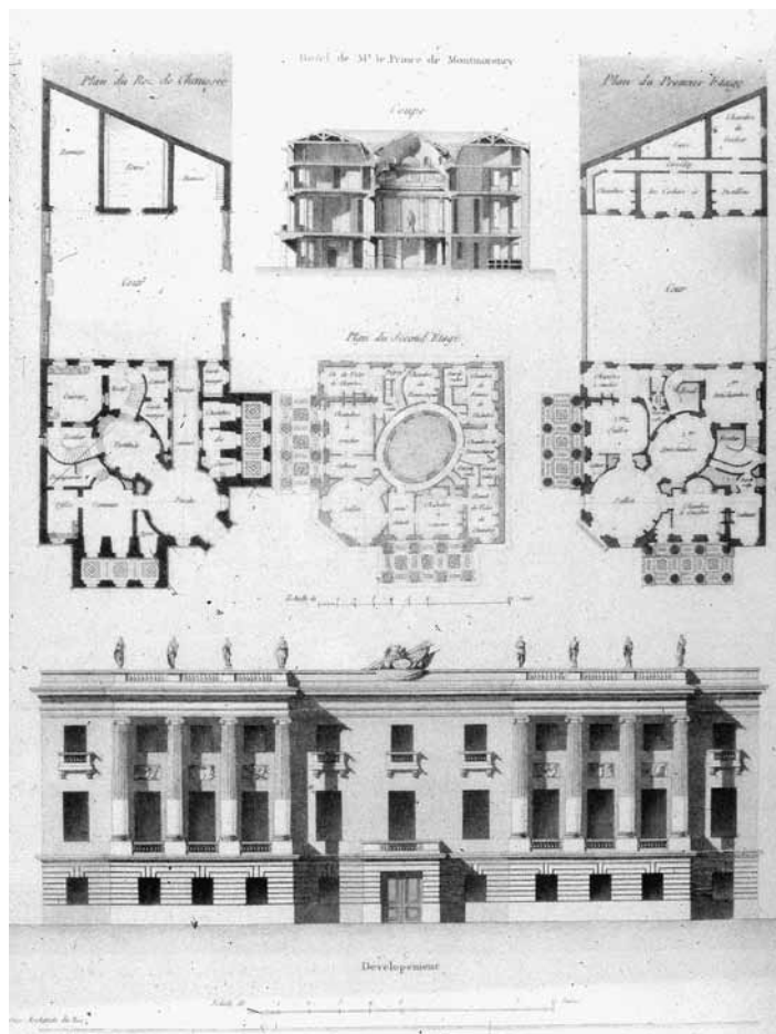
FIG. 6 : CLAUDE NICOLAS LEDOUX, HÔTEL DE MONTMORENCY, CHAUSSEE D'ANTIN, PARIS, 1769. PLAN DU REZ-DE-CHAUSSEE, COUPE, PLAN DU DEUXIÈME ÉTAGE, PLAN DU PREMIER ÉTAGE, ÉLEVATION DE LA FAÇADE PRINCIPALE.
