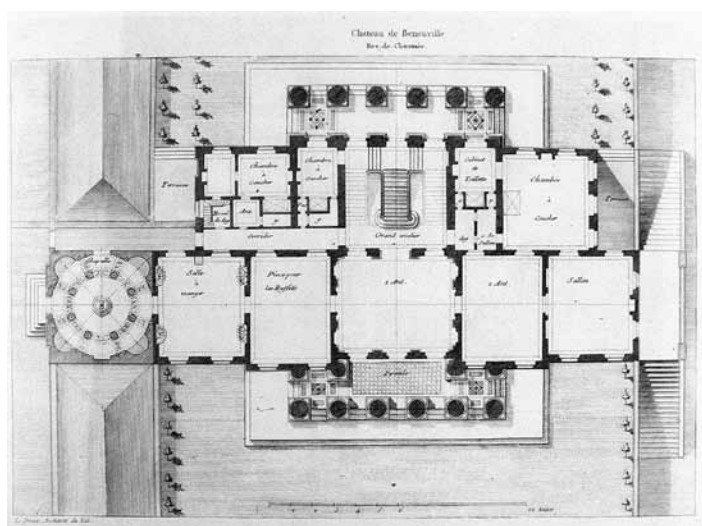
FIG. 7 : CLAUDE NICOLAS LEDOUX, CHÂTEAU DE BÉNOUVILLE, NORMANDIE, 1769. PLAN DU REZ-DE-CHAUSSEE.
