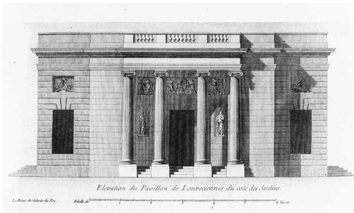
FIG. 8 : CLAUDE NICOLAS LEDOUX, PAVILLON DE MADAME DU BARRY, LOUVECIENNES, 1771. ÉLEVATION DE LA FAÇADE SUR LE JARDIN.
